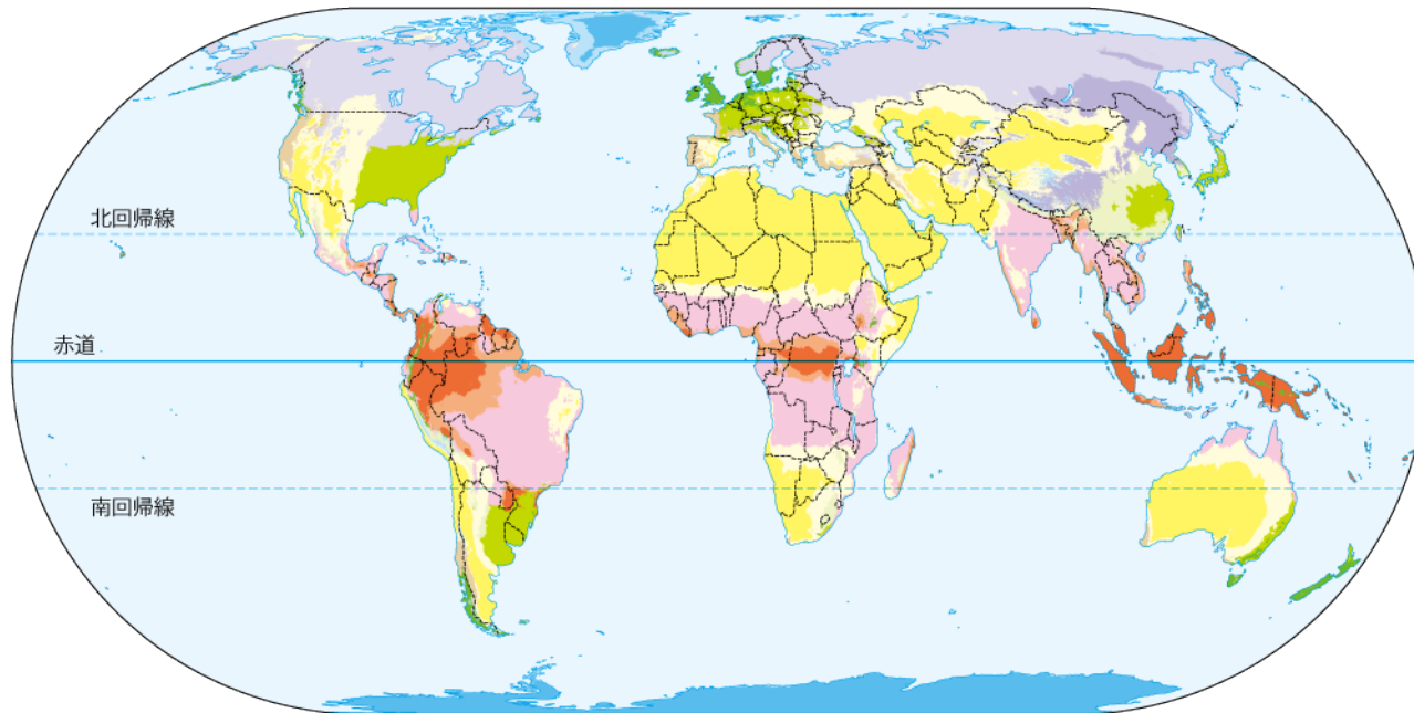
ケッペンの気候区分図(2100年※)
