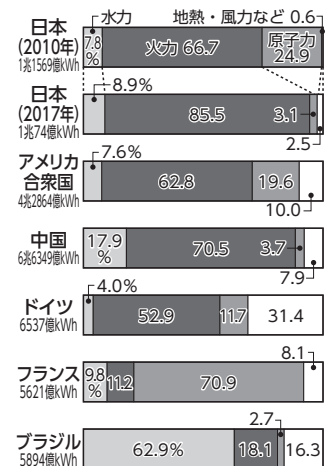
資料Ⅲ 主な国の発電量の内訳
