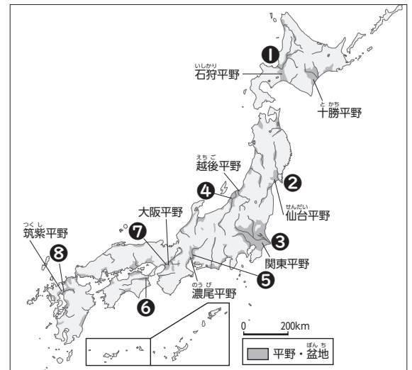
資料Ⅰ 日本の主な川と平野・盆地の分布
