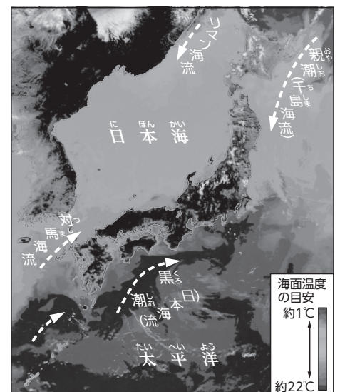
資料Ⅶ 日本周辺の海流
