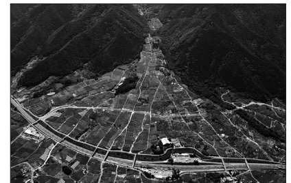
資料Ⅱ 扇状地
